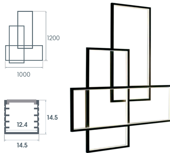
Світильник світлодіодний настінний «ТPIO/ТЕТРА» 220V 126,7W 6480lm (1000х500)х3 та (400х650)х3 чорний корпус
