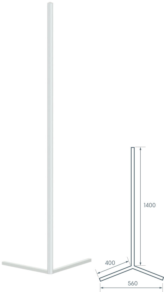
Світильник світлодіодний кутовий підлоговий 220V 12W 1512Lm 1400мм білий корпус
