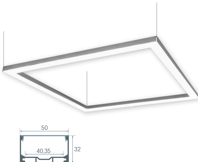
Світильник світлодіодний підвісний «КВАДРА» квадрат 110-240V 108,8W 17300lm 1000x1000
