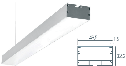
Світильник світлодіодний підвісний лінійний N23-1
