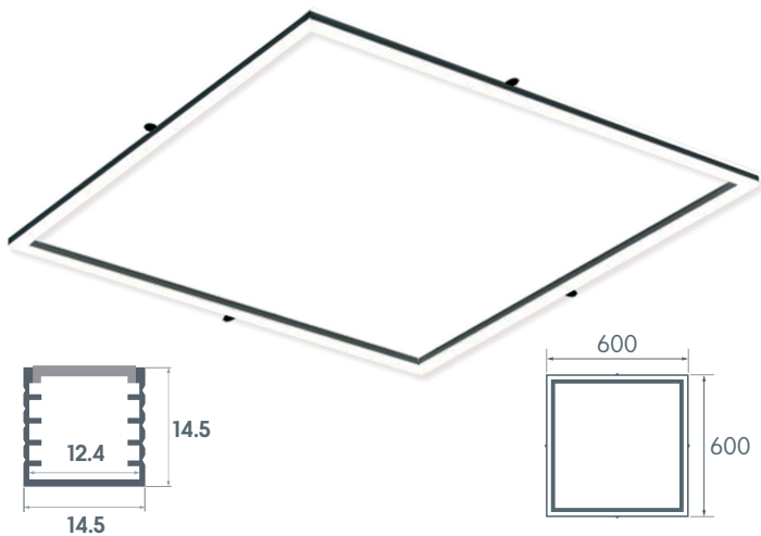
Світильник світлодіодний рамка N4-1 600x600 18W
