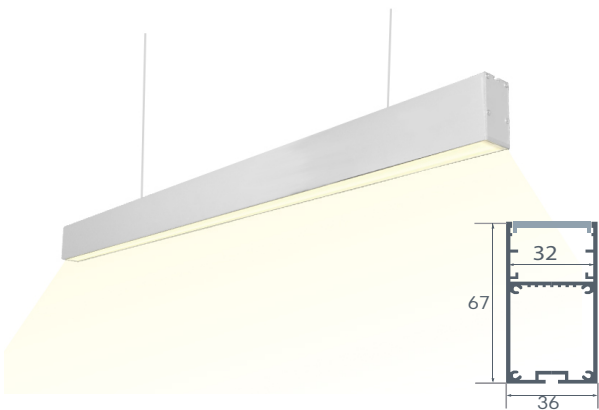
Світильник світлодіодний підвісний лінійний анодований з драйвером (всередині) N44
