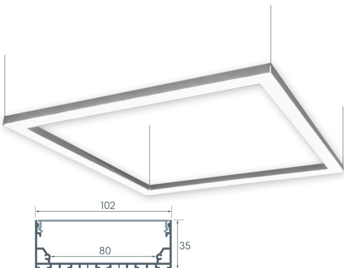
Світильник світлодіодний підвісний «КВАДРА» квадрат 110-240V 163W 25920lm 1000x1000
