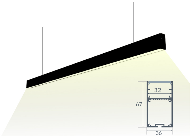
Світильник світлодіодний підвісний лінійний анодований з драйвером (всередині) N44 чорний корпус
