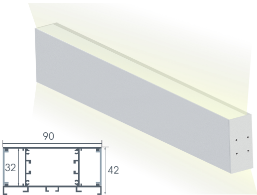
Світильник світлодіодний настінний накладний анодований N39
