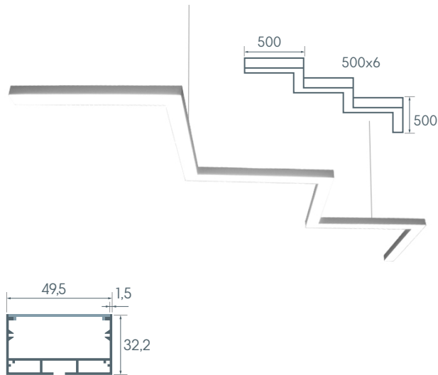
Світильник світлодіодний підвісний «ЛЕВІН-1» 110-240V 57,7W 10800Lm 500x6
