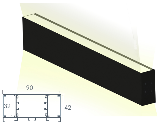
Світильник світлодіодний настінний накладний N39/ чорний корпус
