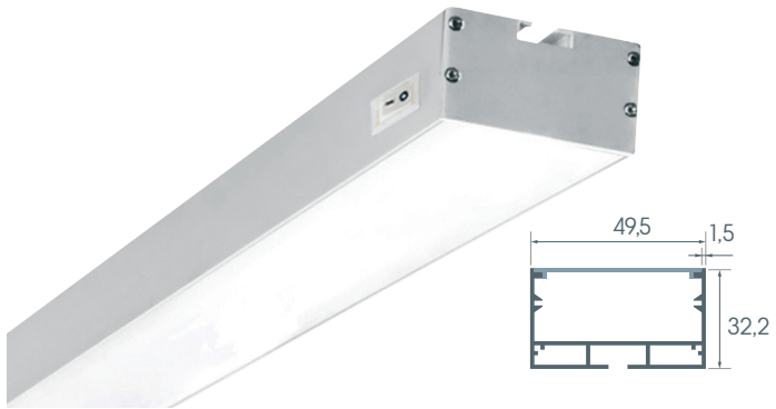
Світильник світлодіодний накладний лінійний «N23-1-500» 220V 9,6W 1800 lm вимикач прямокутний білий
