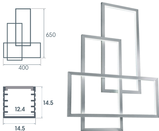
Світильник світлодіодний настінний «ТPIO» 12V, 400х650 анодований корпус 32W
